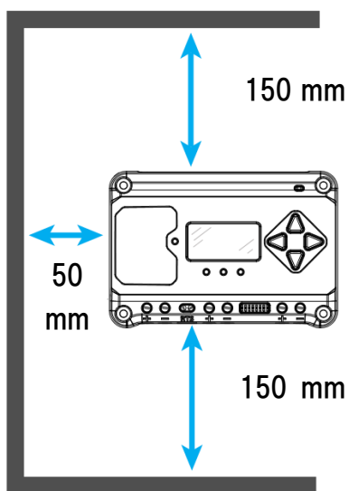
図 3.1 取り付け間隔
