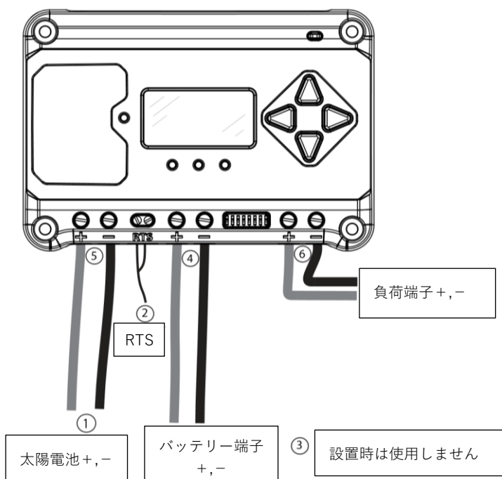
図 3.2 EcoPulse 配線図
